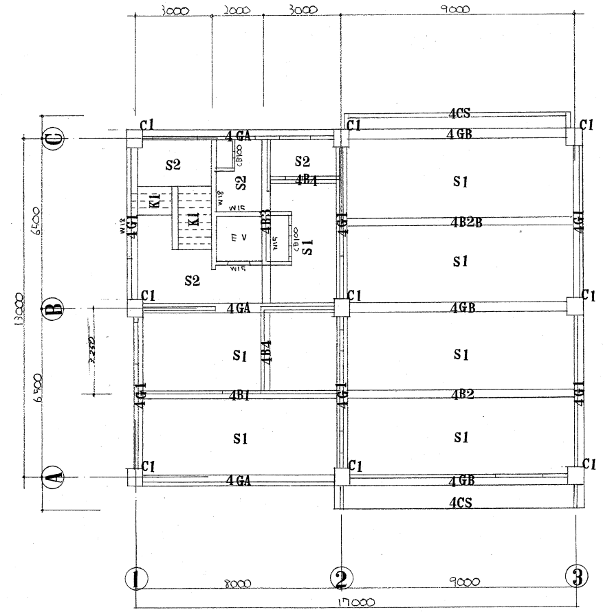
3 階柱壁4階梁伏図 1/100
