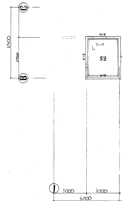
PH室 1/100
