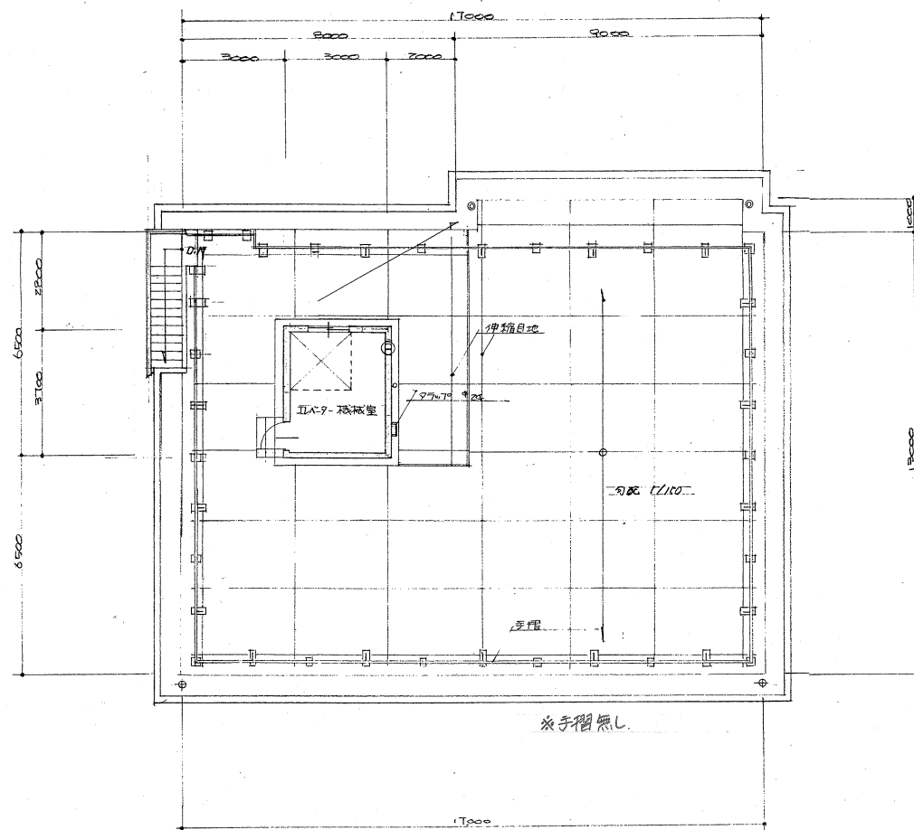
R 1 階 平 面 図 S = 1 : 100
