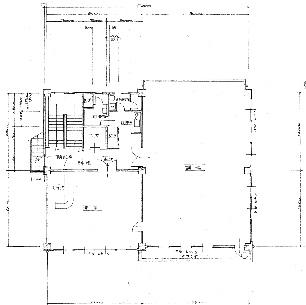
4 階 平 面 図 S = 1 : 100
