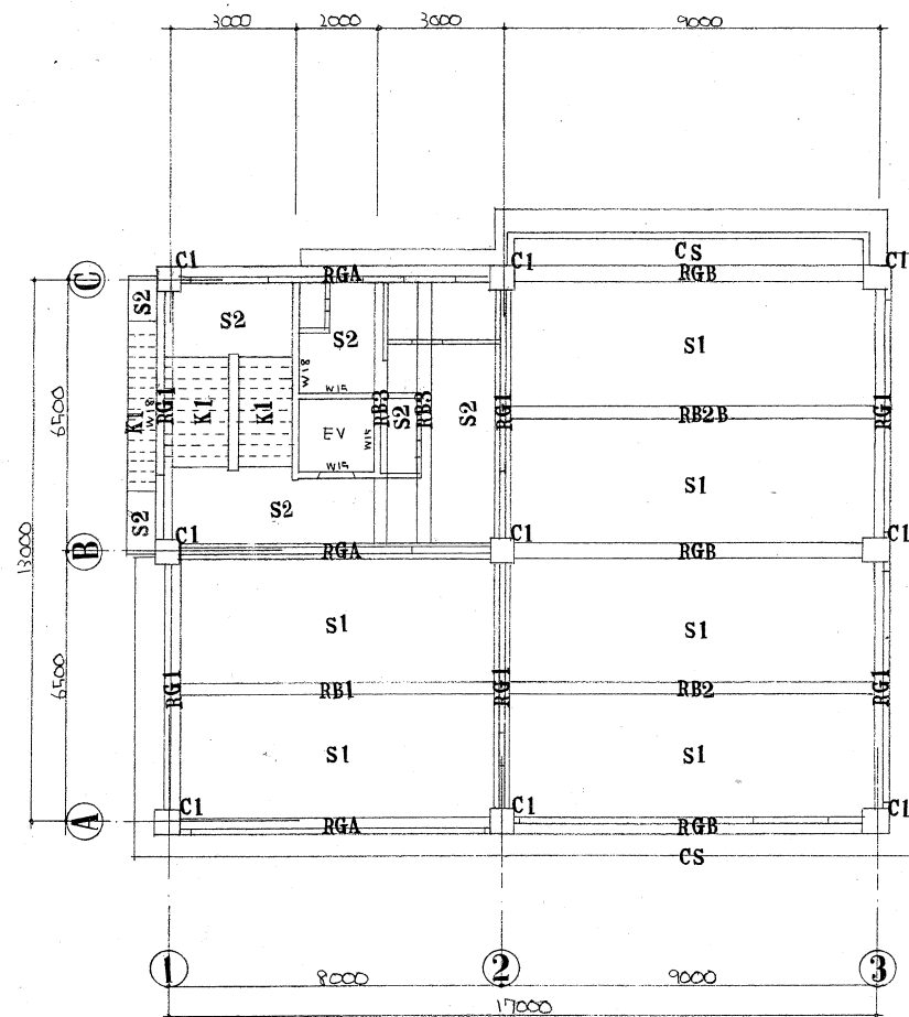
4階花房R階要図 1/100
