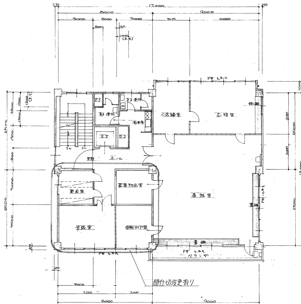
3 階 平 面 図 S = 1 : 100
