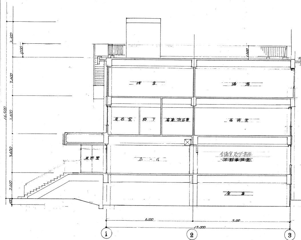
東西断面図
