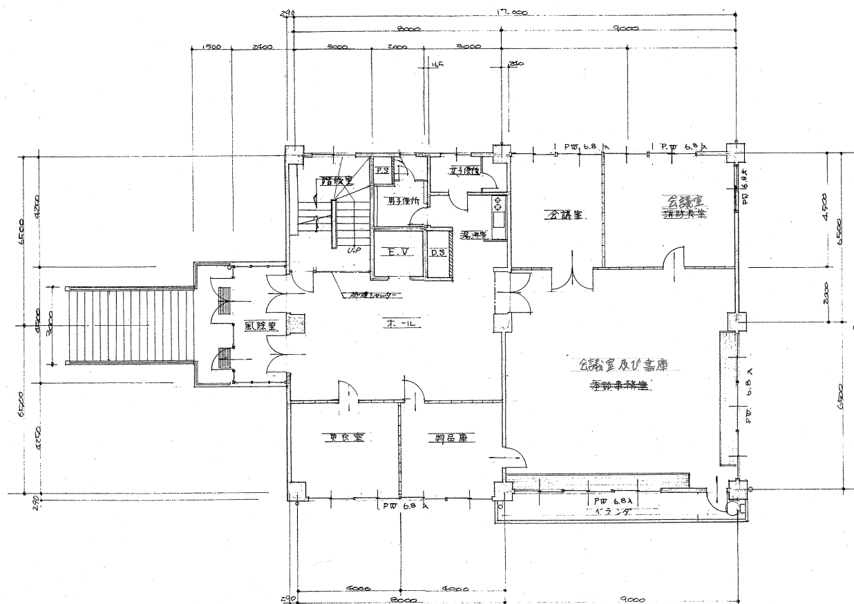
2 階 平 面 図 8 = 1 : 100
