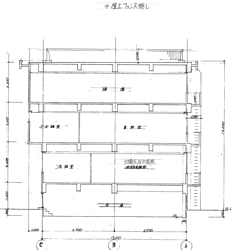
南北断面図
