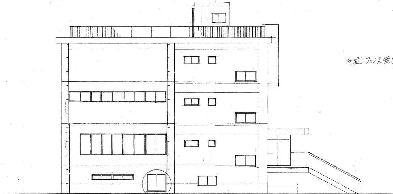
北側立面図
