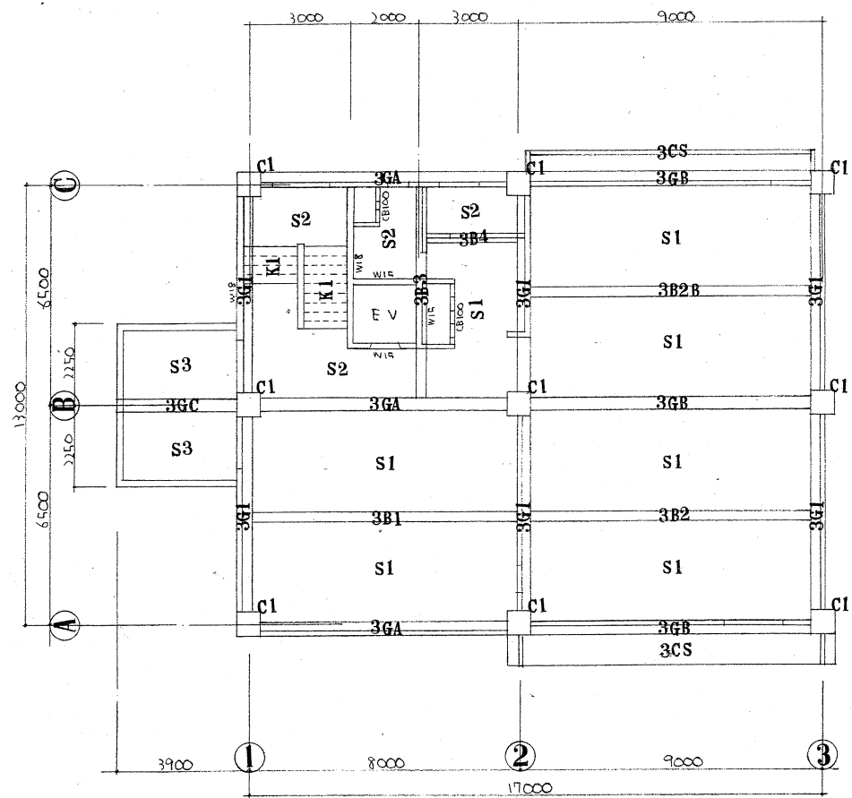
2 階柱壁3階梁伏図 1/100
